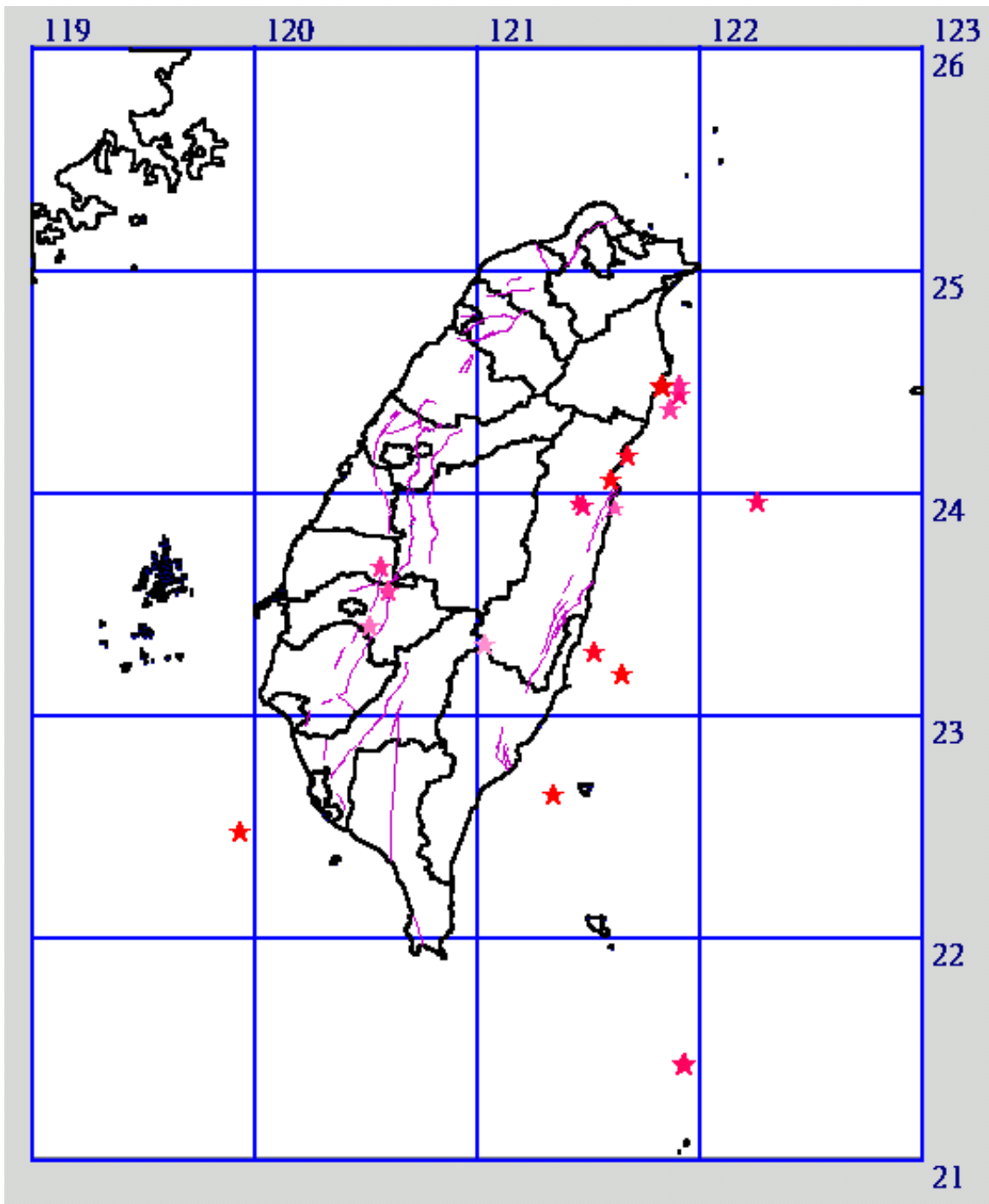
圖二、2002年12月有感地震震央分佈圖。
