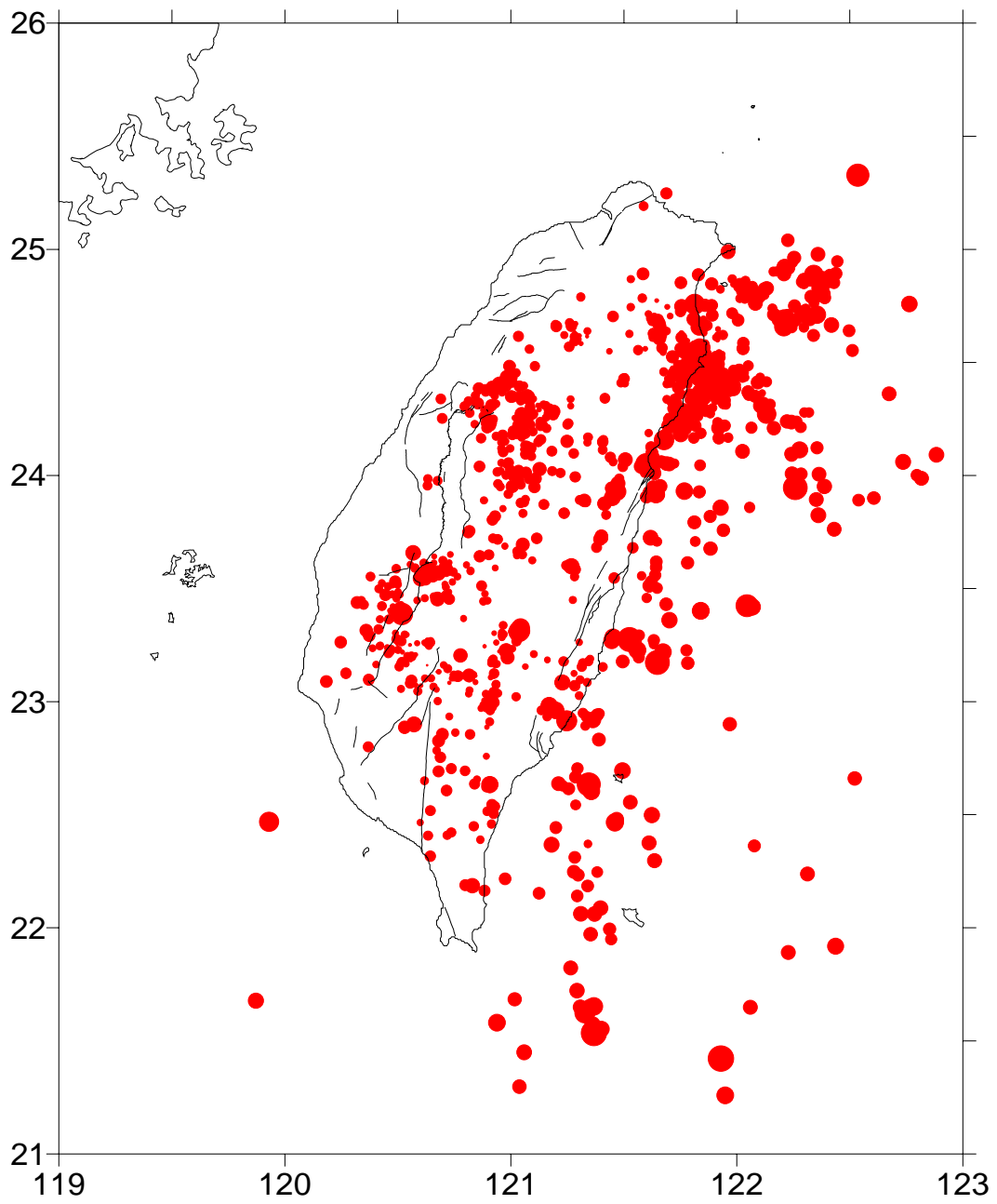
圖一、2002 年 12 月份地震震央分佈圖。
