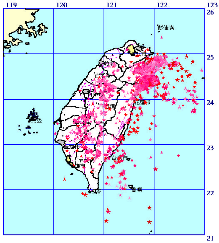
圖一、2002 年五月（完整處理 20 天）地震震央分佈圖
