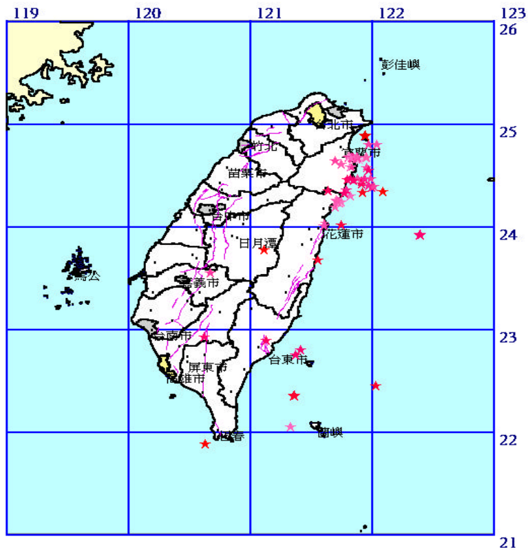
圖二、2002 年五月有感地震震央分佈圖
